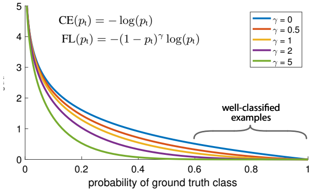
图1. 我们提出了一种新颖的损失函数，称为Focal Loss，它在标准交叉熵准则中增加了一个因子 (1 - p_t)^\gamma 。设定 \gamma > 0 会降低分类良好样本 ( p_t > .5 ) 的相对损失，从而更关注难以分类的错误样本。如实验所示，所提出的焦点损失能够在存在大量简单背景样本的情况下，训练出高精度的密集目标检测器。
